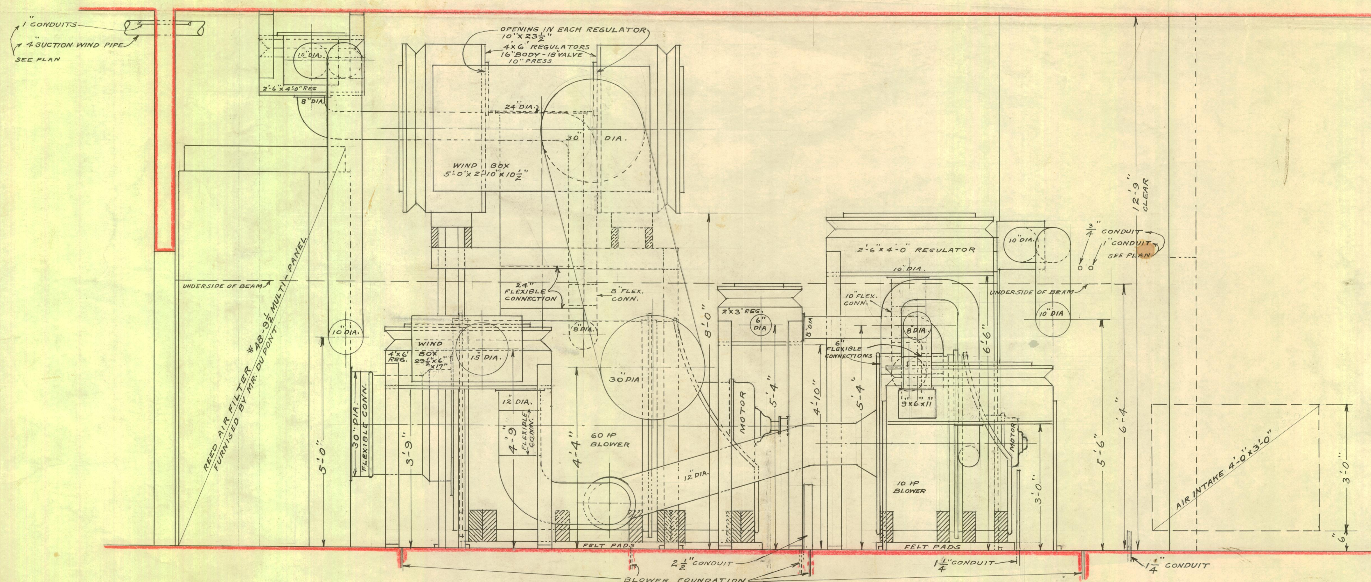
ELEVATION
